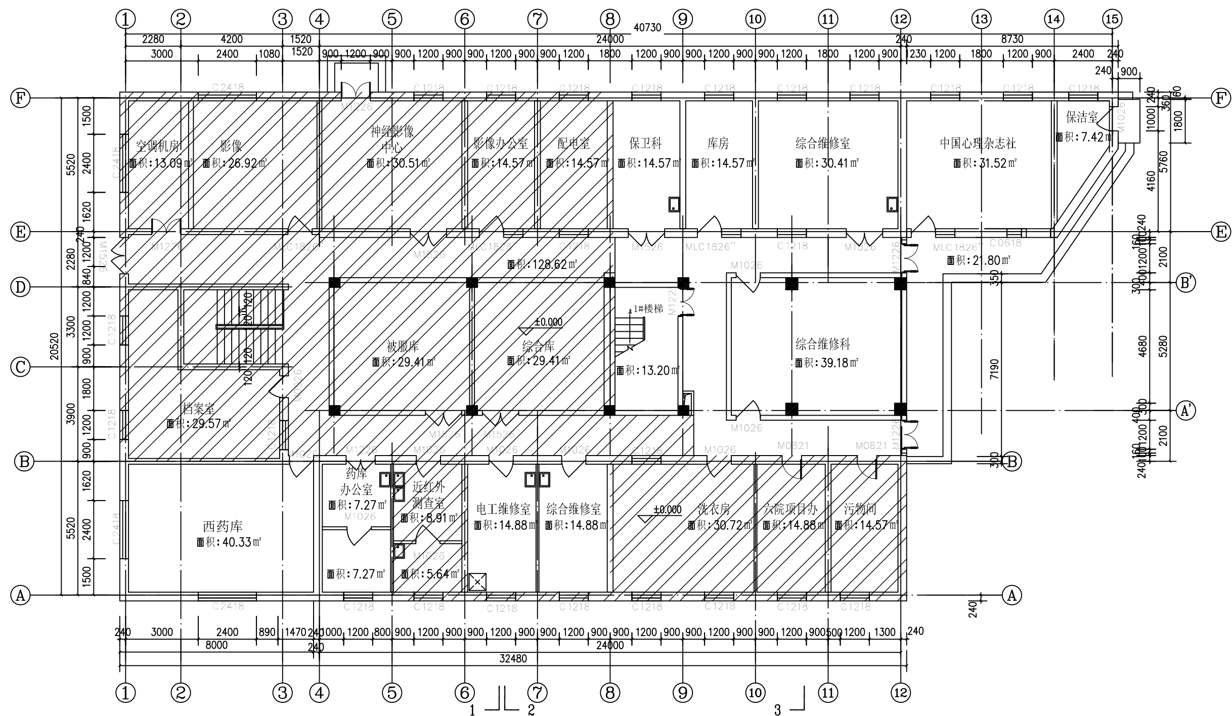
一层平面图 1:100
